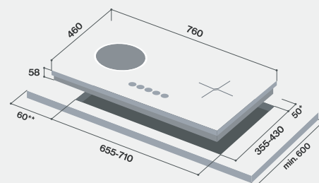
RB-7152HEF-ZB
