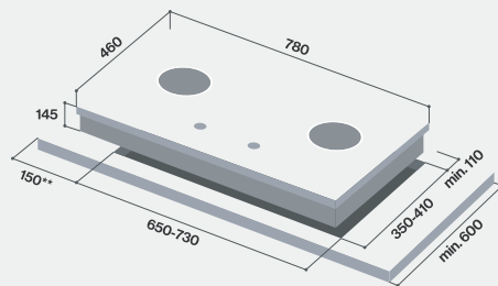
RB-38HS
