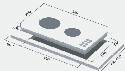
RB-5022E-CB
