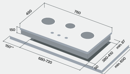
RB-27HS
