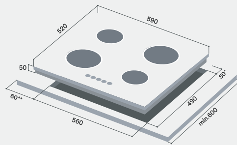
RB-5022E-CB
