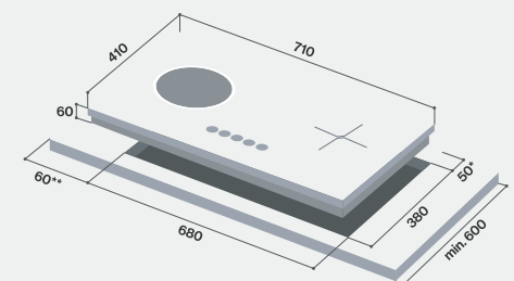
RB-7022HE-CB
