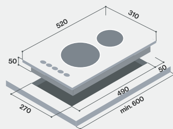
RB-3012E-CB
