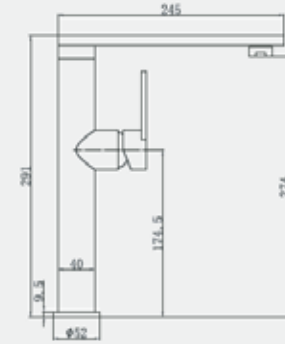
SMB-01B
