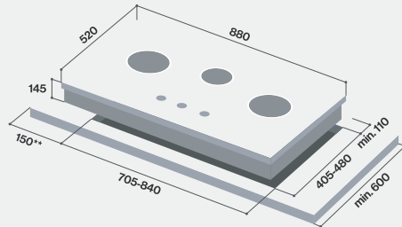
RB-982G
